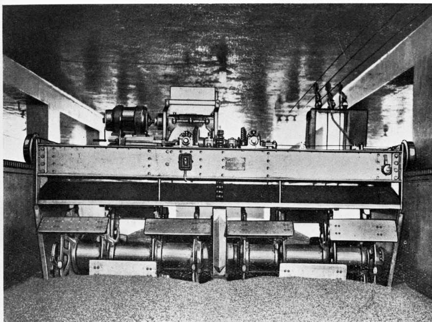
GERMINATION DU GRAIN (RETOURNEUR)
