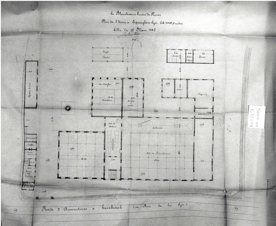
Blanchisserie linière de France. Plan au sol, 1882 (AD Nord ; M4172456).
