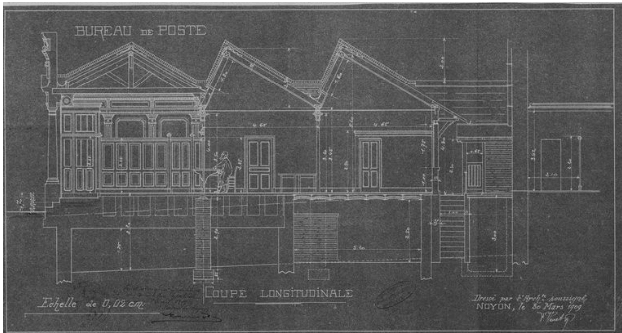
Coupe longitudinale, par Venet, 1909 (AD Oise ; série O).
