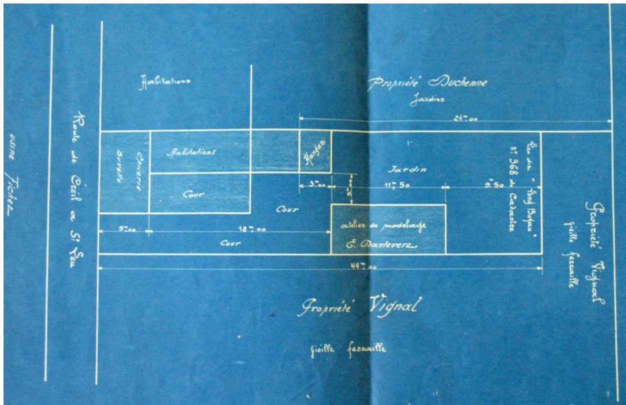
Plan de l'atelier de menuiserie, 1924 (AD Oise ; 5Mp2454/2).
