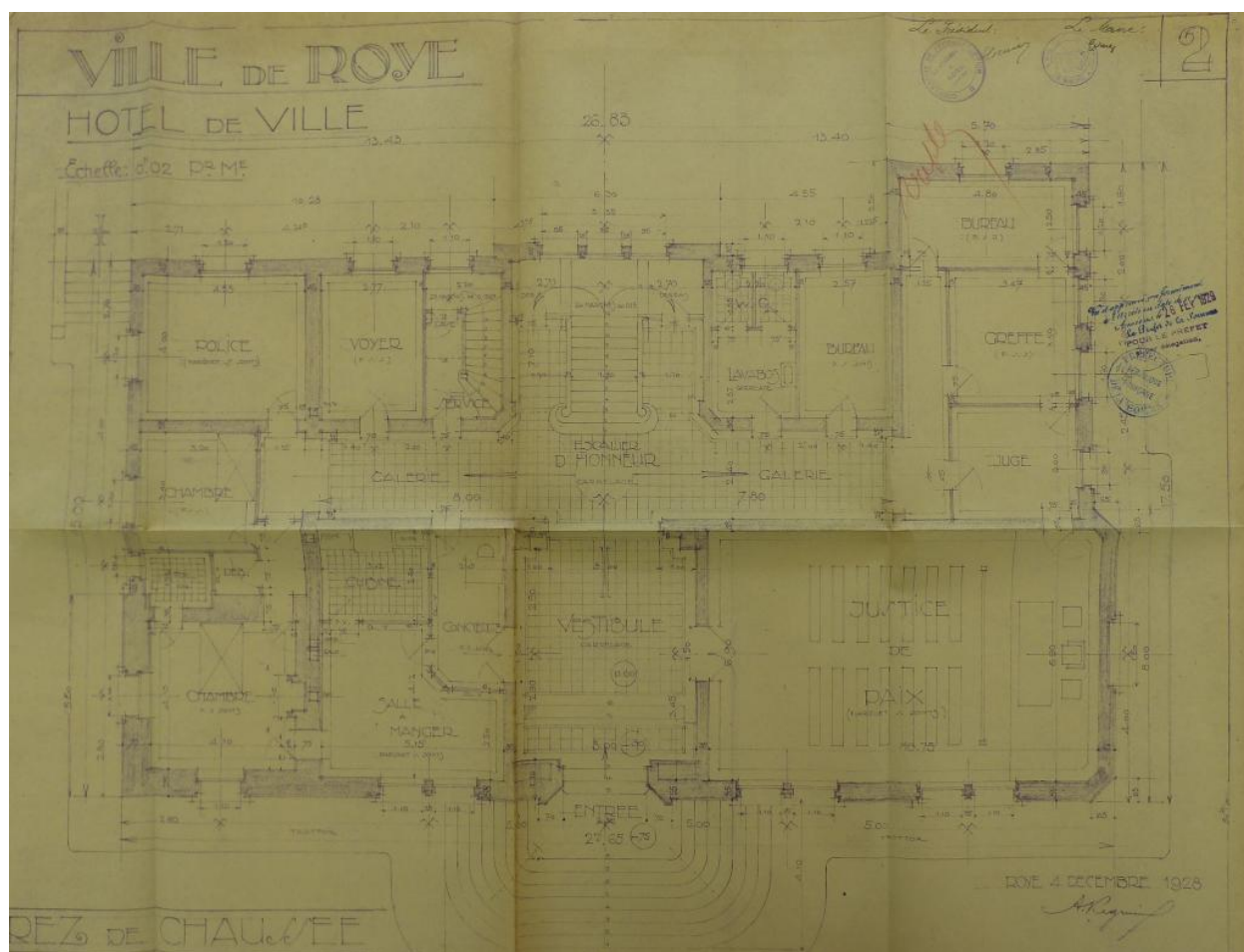
Ville de Roye. Hôtel de ville. Plan du rez-de-chaussée. A. Régnier architecte, 1928 (AD Somme ; 99O 3296).
