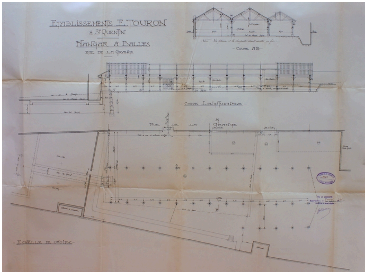
Plans du hangar à balles de coton, par Nalet (arch.), 1926 (AC Saint-Quentin).
