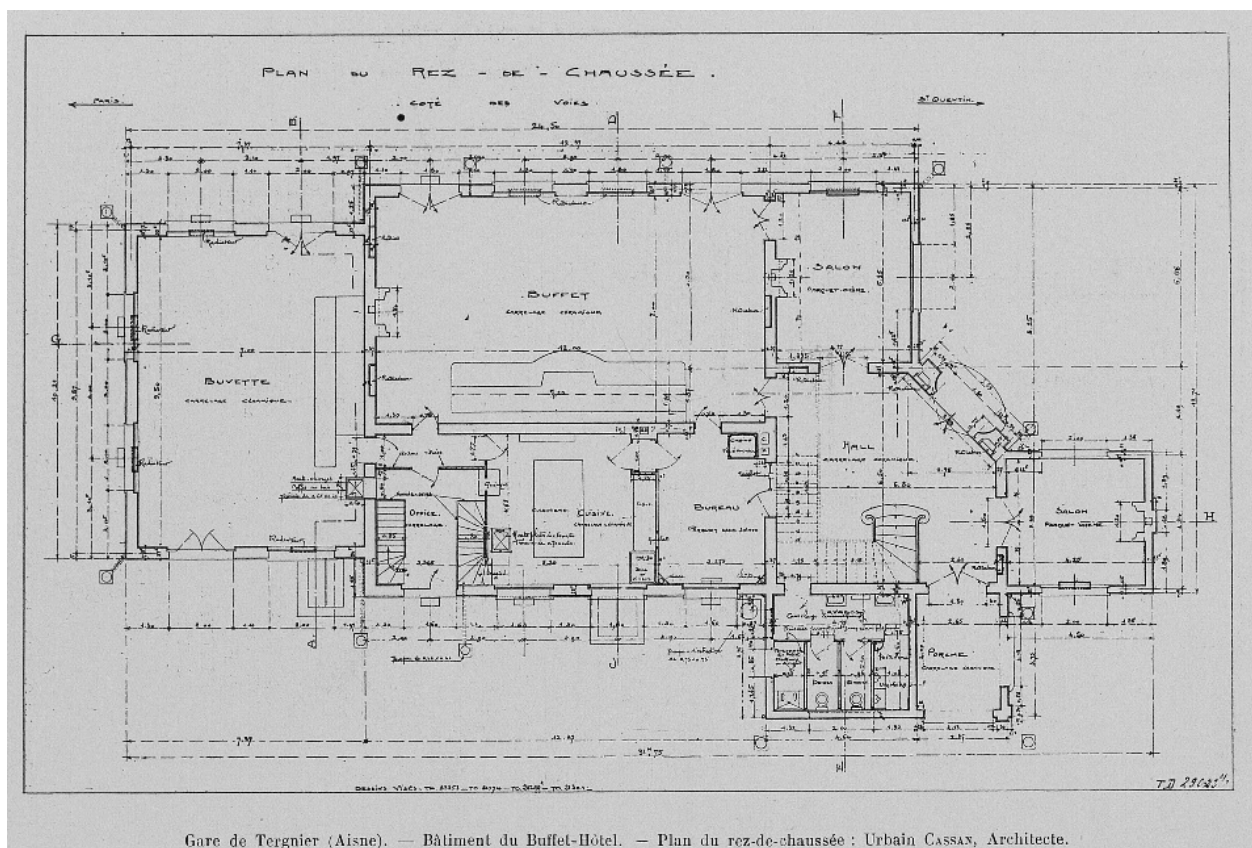
Gare de Tergnier (Aisne). — Bâtiment du Buffet-Hôtel. — Plan du rez-de-chaussée : Urbain CASSAN, Architecte.
