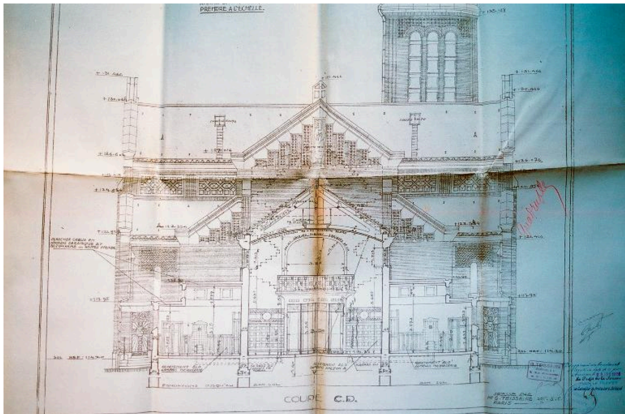
Coupe transversale, 3e projet de reconstruction par Teisseire, 28 juin 1926 (AD Somme ; 99 O 1122).
