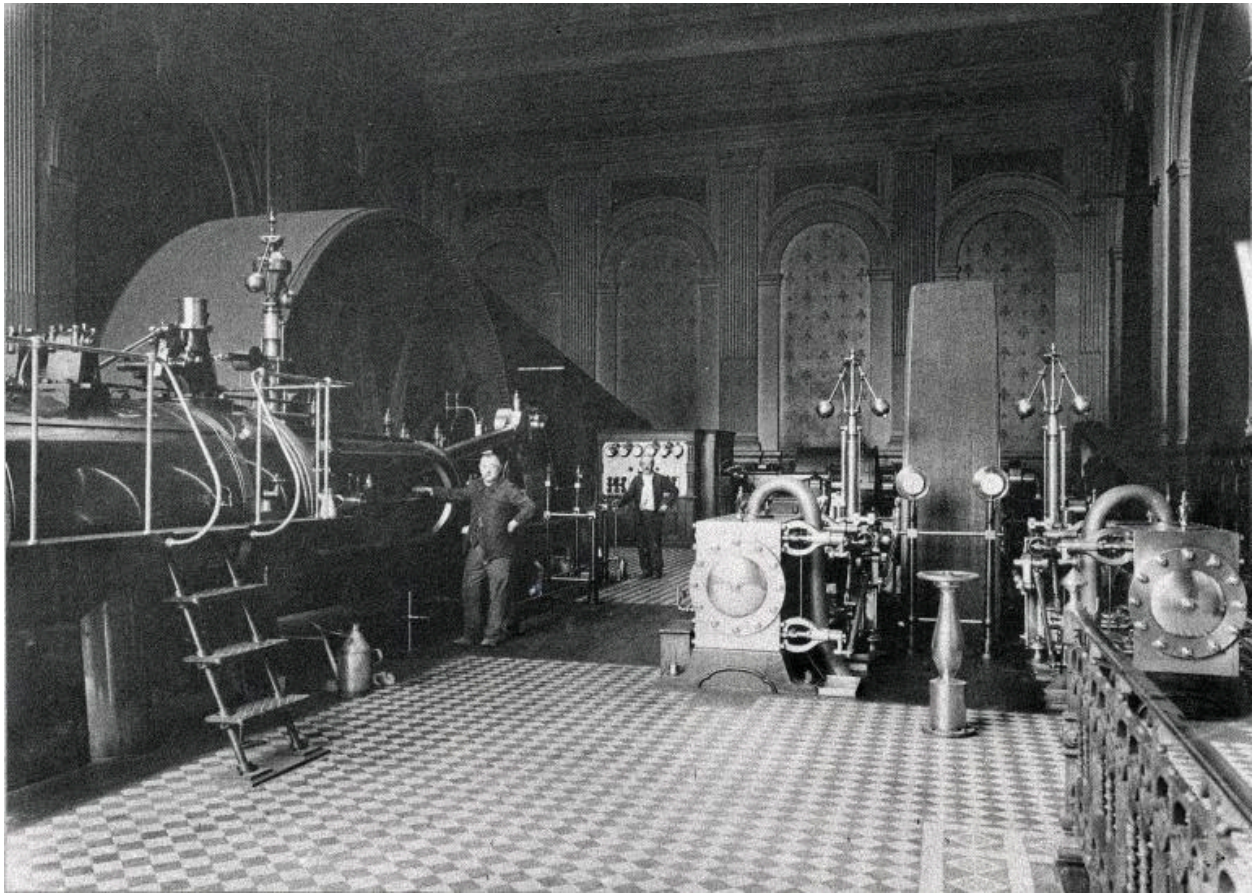
Vue intérieure de la salle des machines et de la machine à vapeur, vers 1900 (AP).
