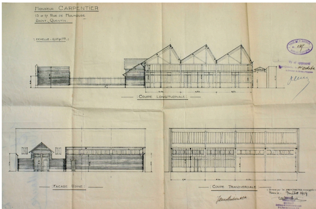
Élévation et coupe des ateliers de l'usine, 1919 (AC Saint-Quentin).
