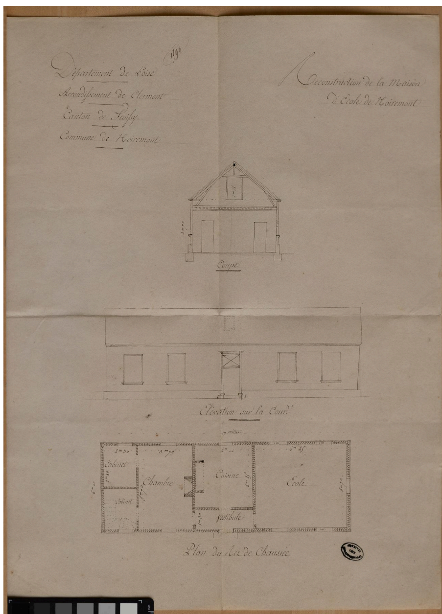
Plan pour la reconstruction de la maison d'école de Noirémont, 1840 (AD Oise).
