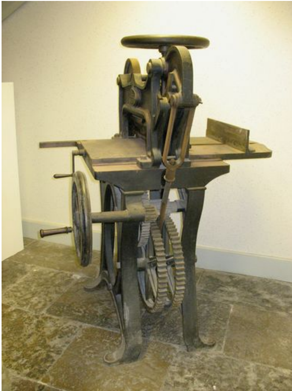
Vue générale : machine la plus petite
