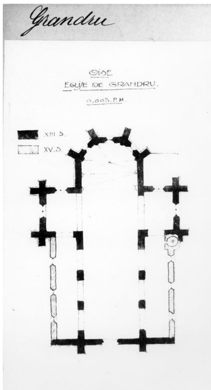
Plan de l'église (Médiathèque du Patrimoine).
