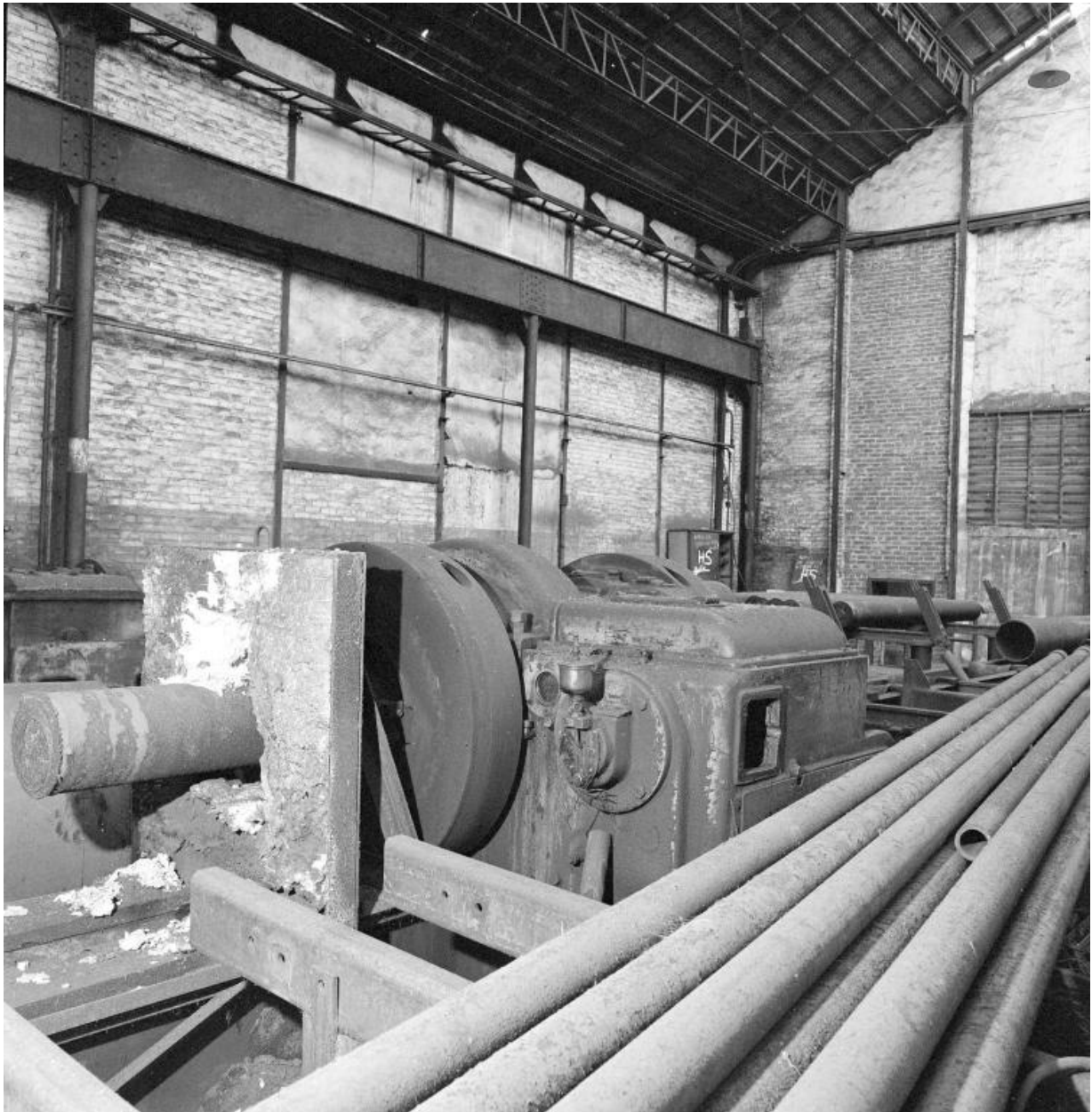
Machine d'étrirage (usine B).
