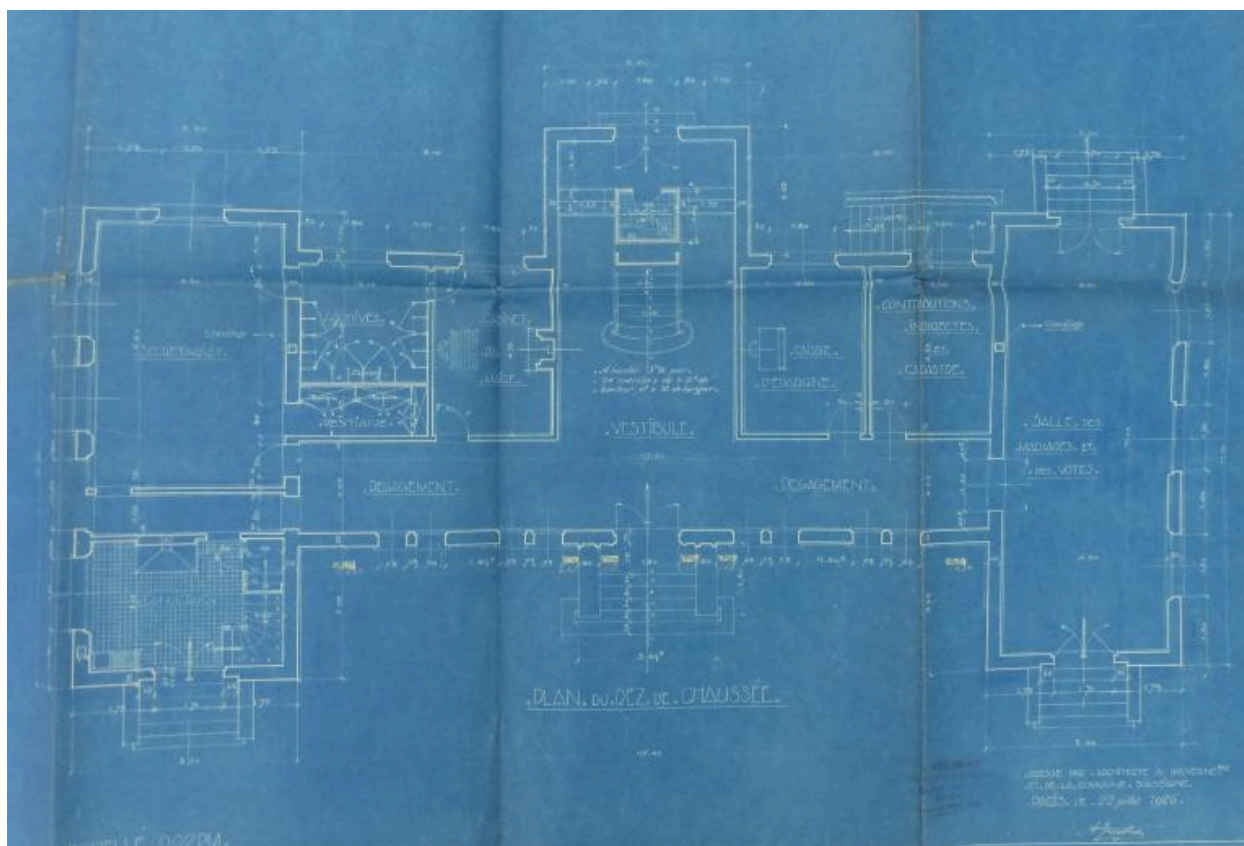
Projet de reconstruction de l'église de Villers-Bretonneux. Somme. Plan du rez-de-chaussée. Tirage de plan, A. Guilbert architecte, 22 juillet 1926 (AD Somme ; 99O 3737).
