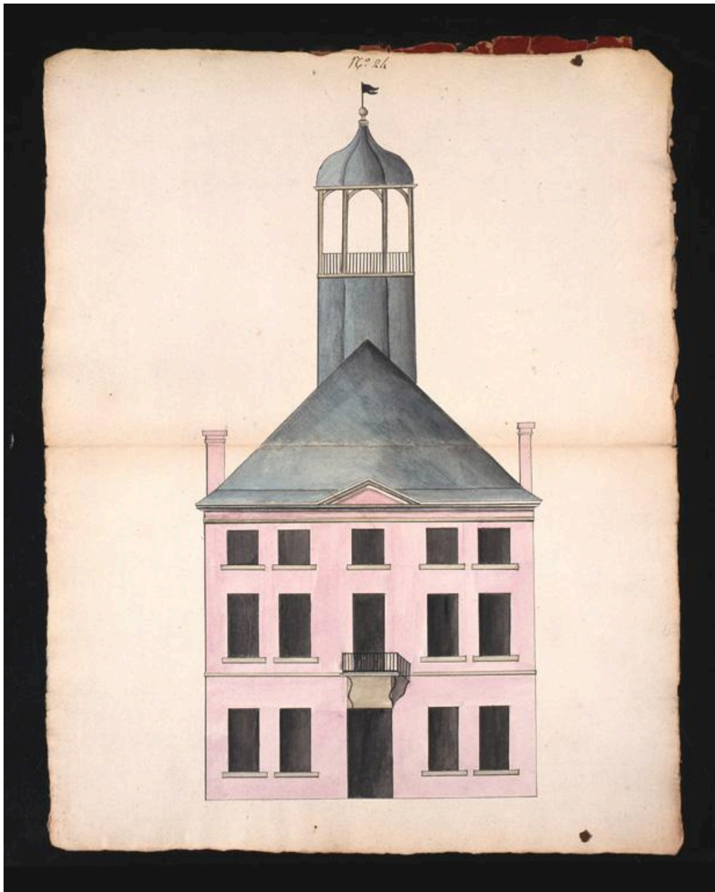
Elévation de la façade principale de l'hôtel de ville de Vervins : projet de réhabilitation non suivi d'exécution, vers 1820.
