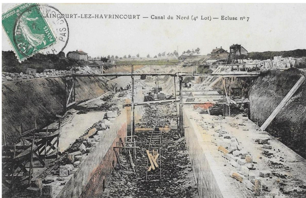
Base des bajoyers en cours de construction (premier niveau de brique et second niveau de bloc de grès), carte postale entre 1908 et 1914 (collection particulière).
