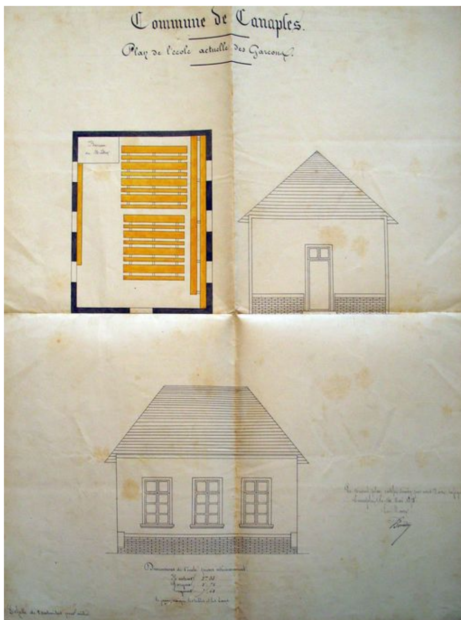
Plan et élévations, 1875 (AD Somme ; 99 O 1024).
