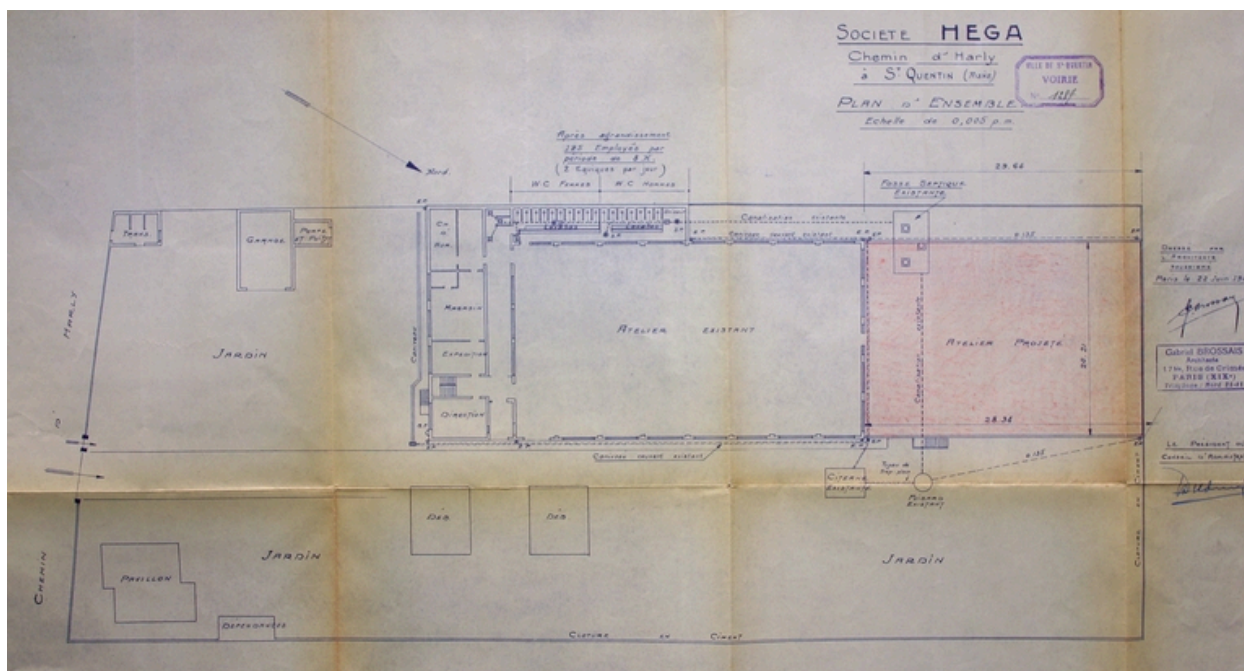
Plan d'ensemble de l'usine, par Brossais, 1946 (AC Saint-Quentin).
