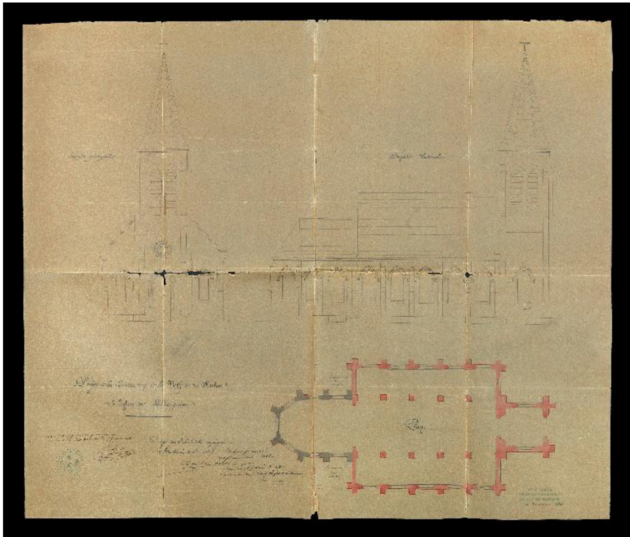
Projet de construction de la nef et du clocher : élévations et plan, par Coulombel, 1859 (AD Somme ; 99 O 1355).
