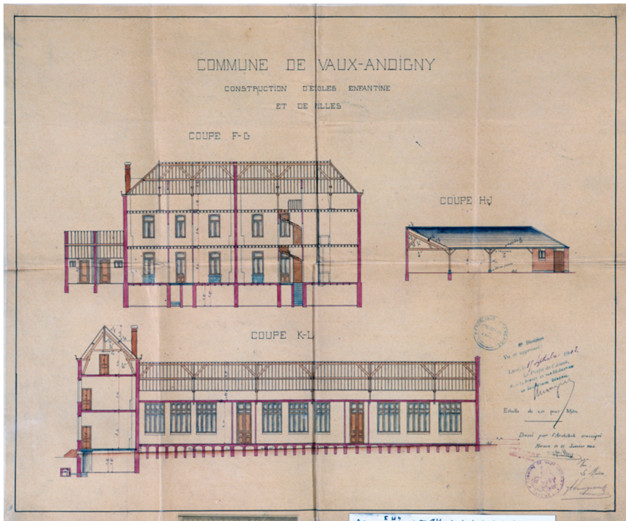
Commune de Vaux-Andigny. Construction d'une école enfantine et de filles. Coupes, Désiré Leroy architecte, 1902 (AD Aisne ; Vaux-Andigny : 4 M 3).
