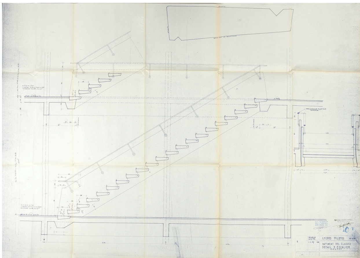
Dessin d'un escalier intérieur du collège de la cité scolaire Yves Kernanec à Marcq en Baroeul, 1958.
