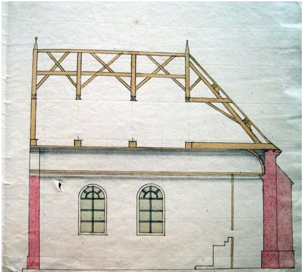
Elévation latérale de l'extension projetée en 1771 (AD Somme ; 4 G 1624).
