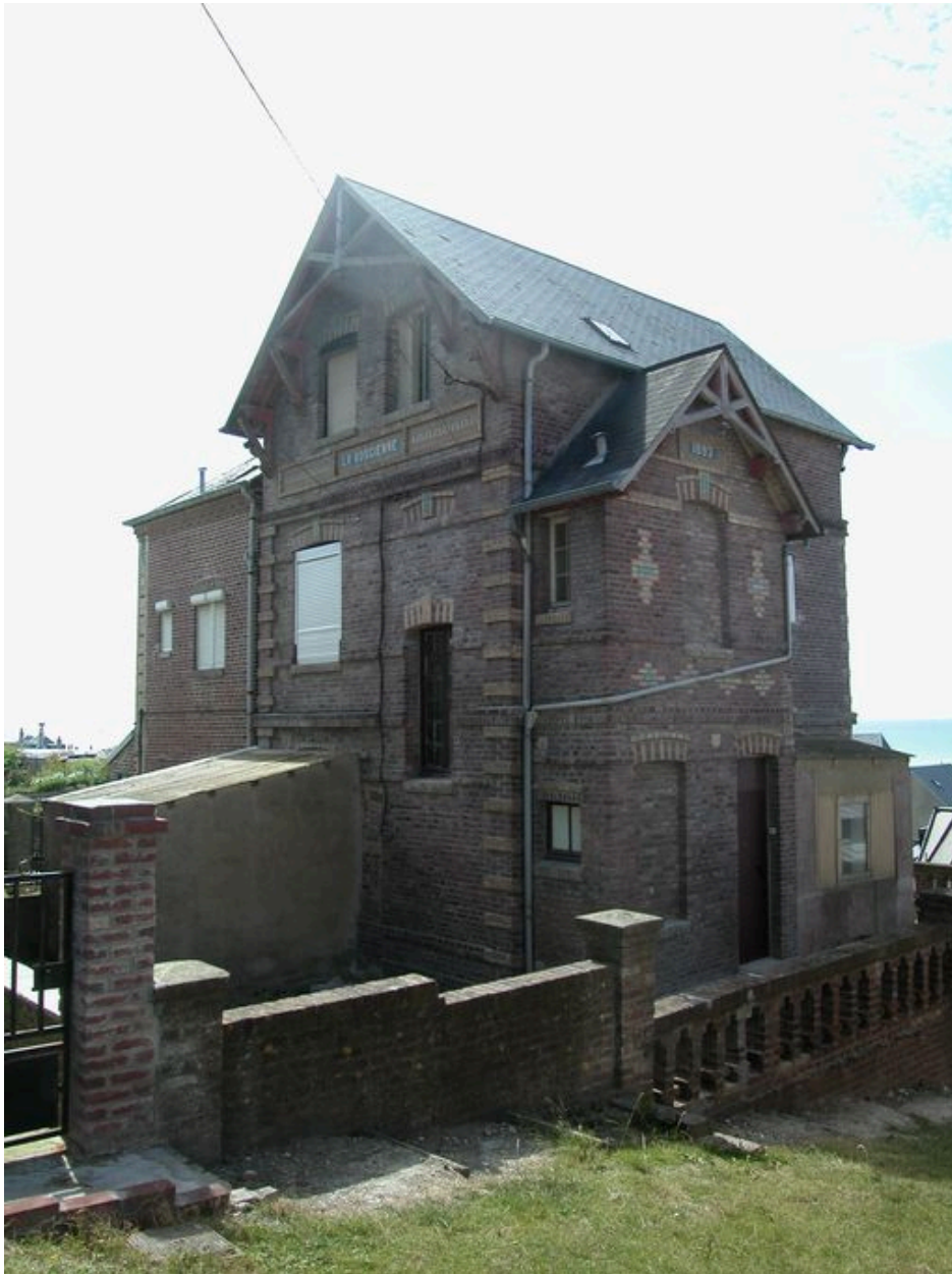
Vue de trois-quarts sur les élévations postérieure et latéral gauche, depuis la rue Dingeon.
