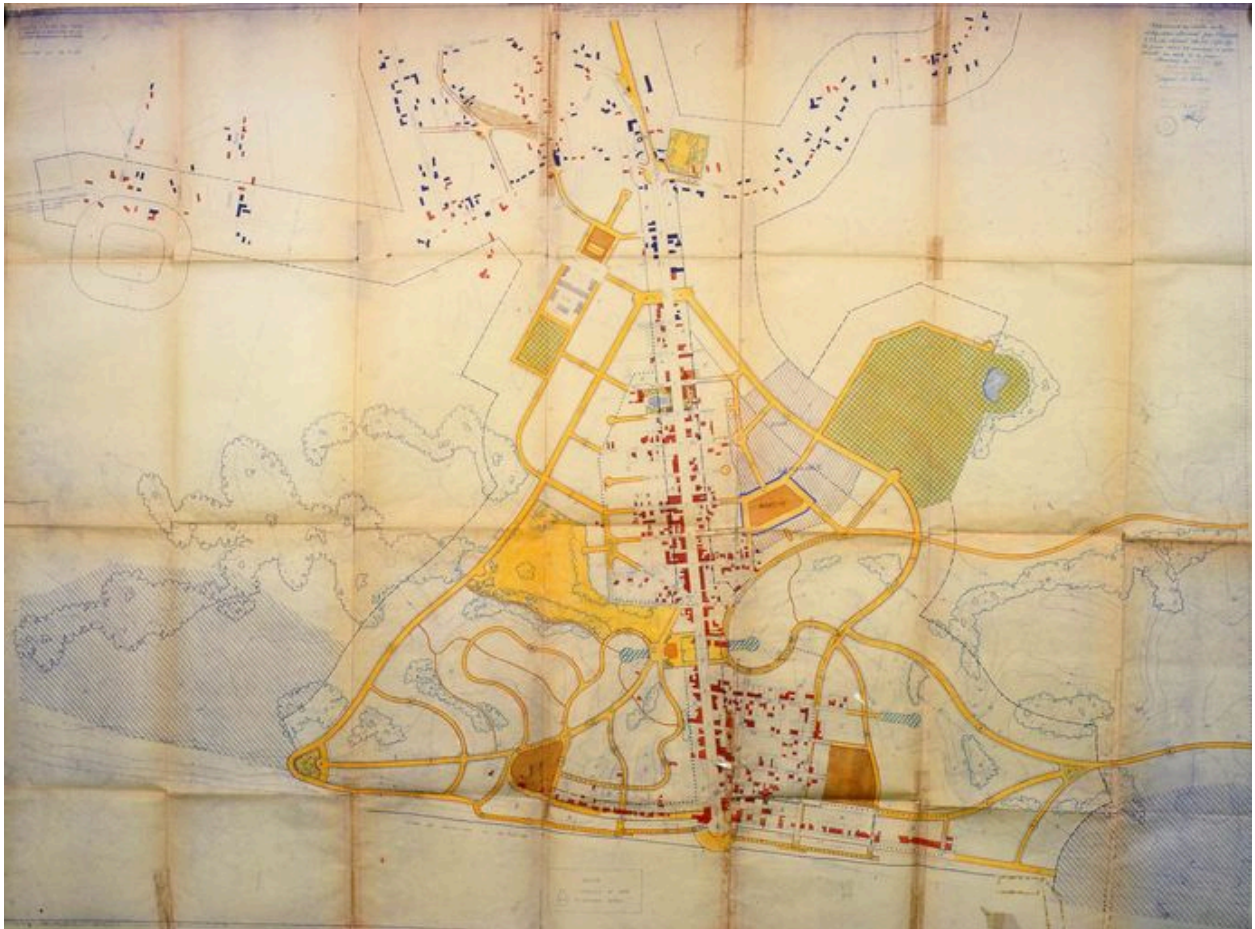
Plan projeté pour la reconstruction de Fort-Mahon-Plage, par G. Lecompte urbaniste, 20 juillet 1947 (AD Somme ; 1102 W 334).
