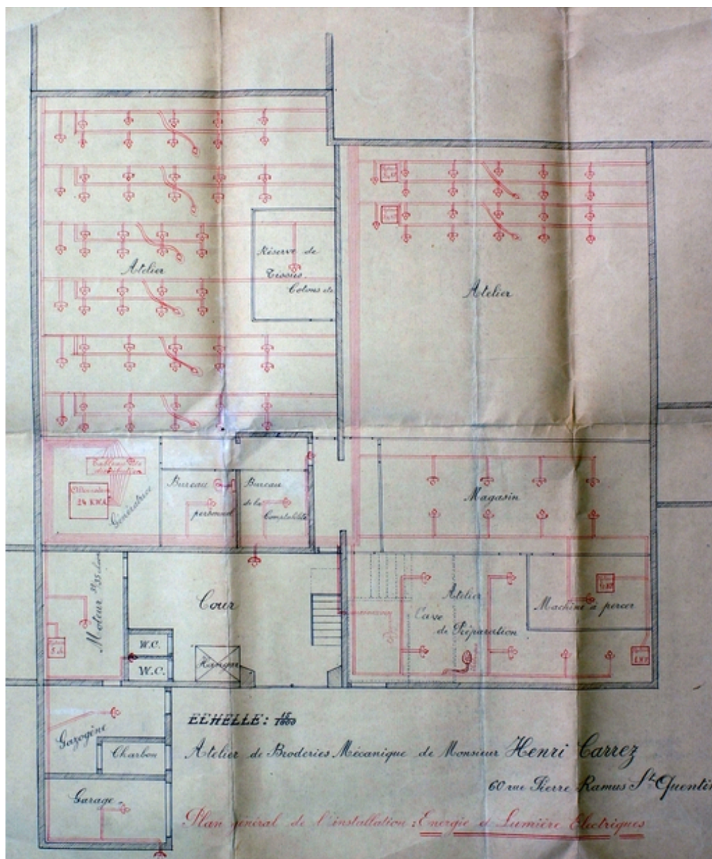
Plan général de l'installation électrique de l'usine à la veille de la Première Guerre mondiale (AD Aisne).
