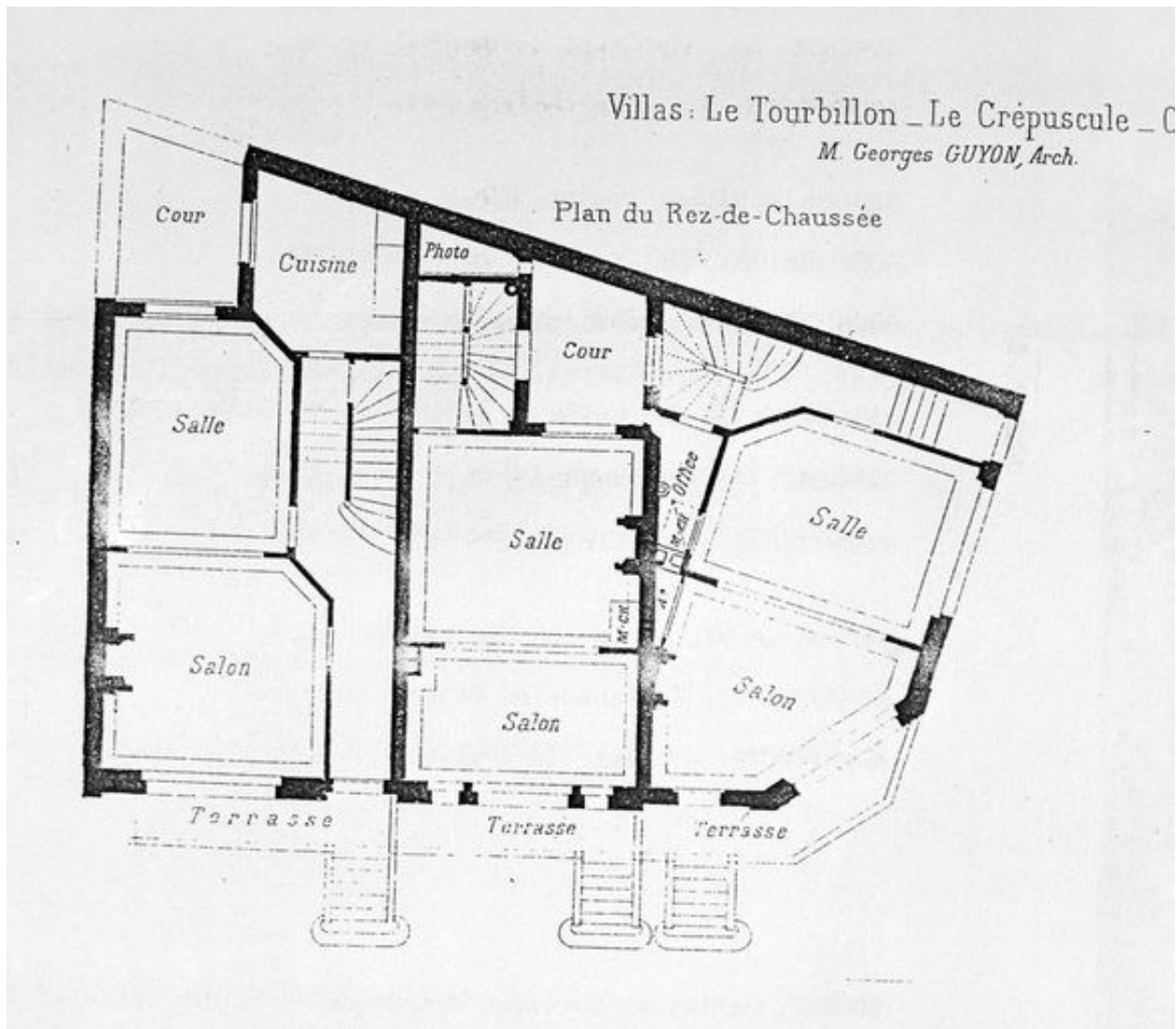
Villas Le Tourbillon, Le Crépuscule, Clair de Lune, plan du rez-de-chaussée.
