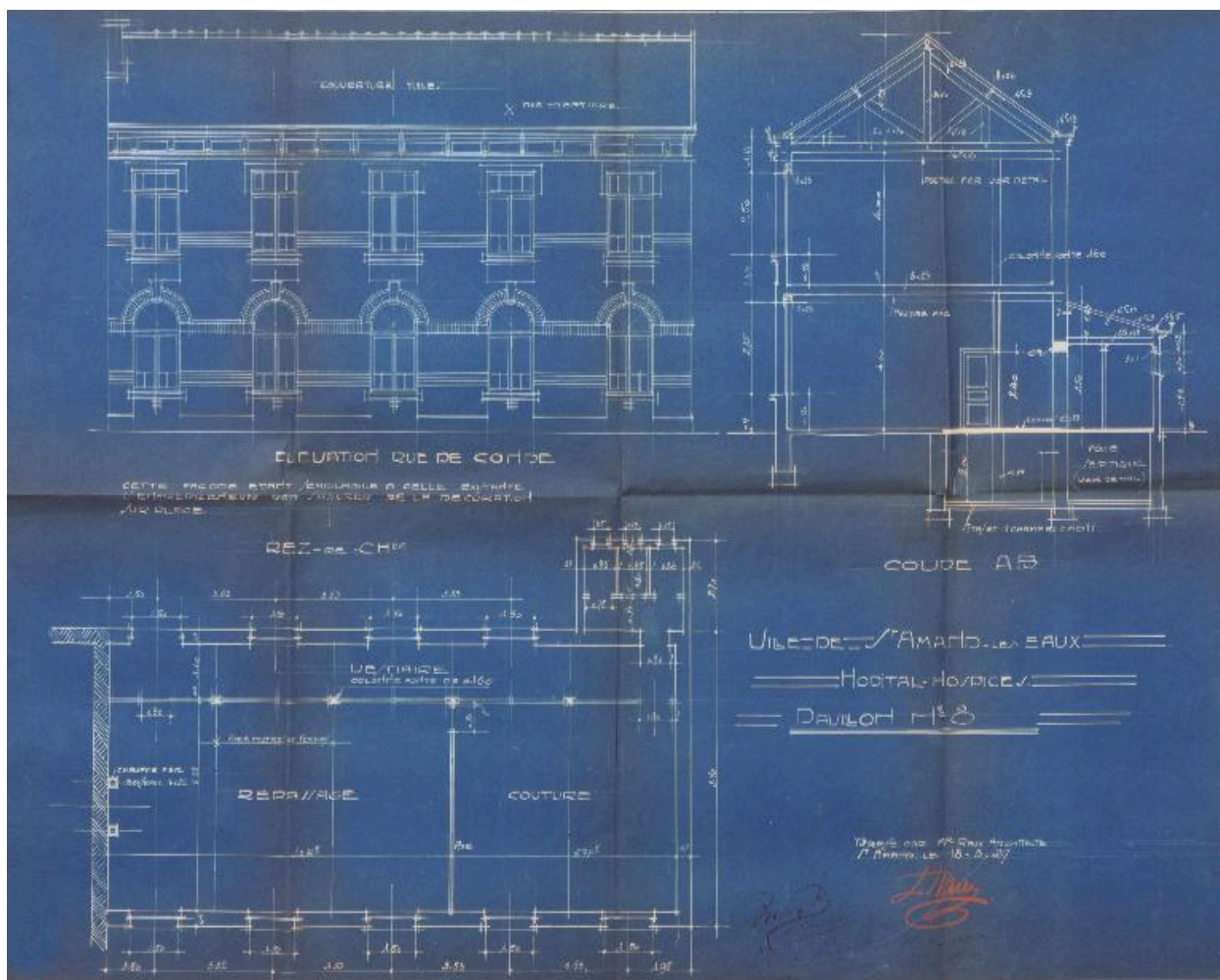
Plan, coupe et élévation du pavillon 8 "ménager", Léon Raux architecte, 1929 (AH, centre hospitalier Saint-Amand-les-Eaux).
