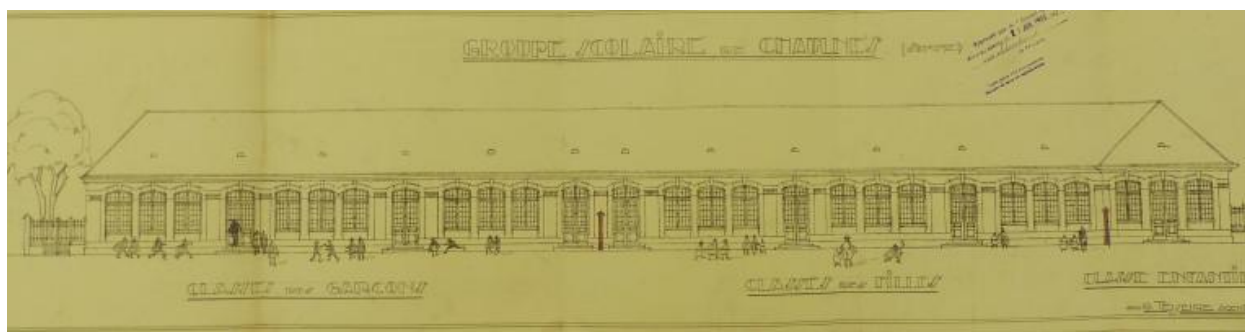
Groupe scolaire de Chaulnes. Projet de reconstruction. Les salles de classe : façades sur la cour (AD Somme ; 10R 308).
