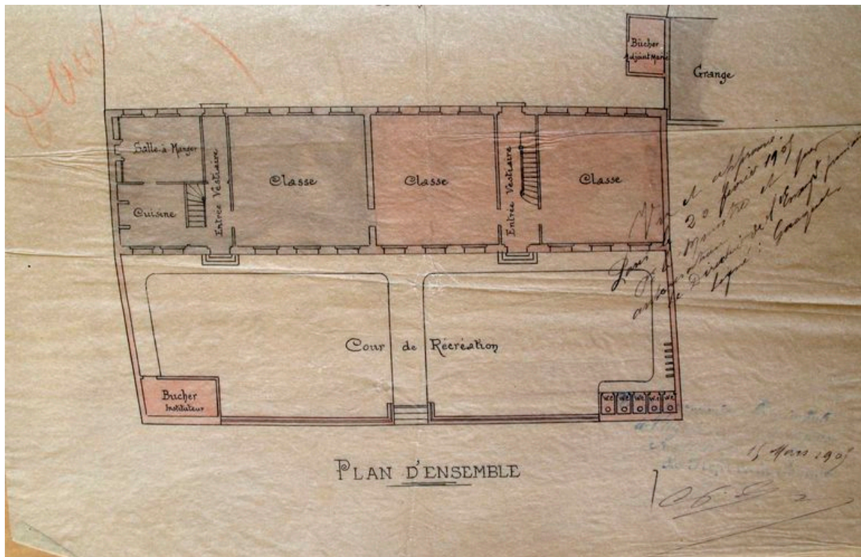
Plan du rez-de-chaussée par Anatole Bienaimé, 1903 (AD Somme ; 99 O 680).
