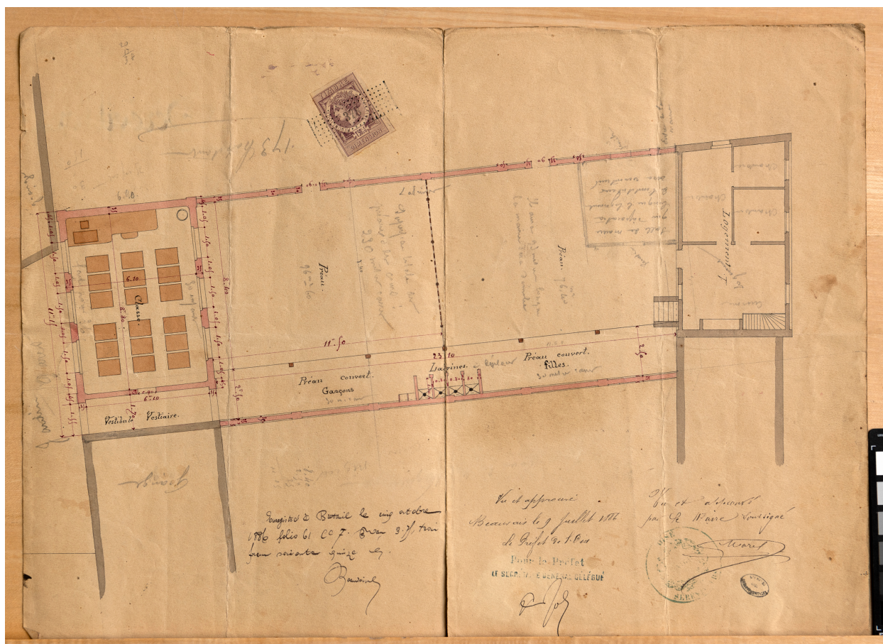
Sérévillers (Oise). Plan du projet d'école avec logement de l'instituteur, 1886 (AD Oise).
