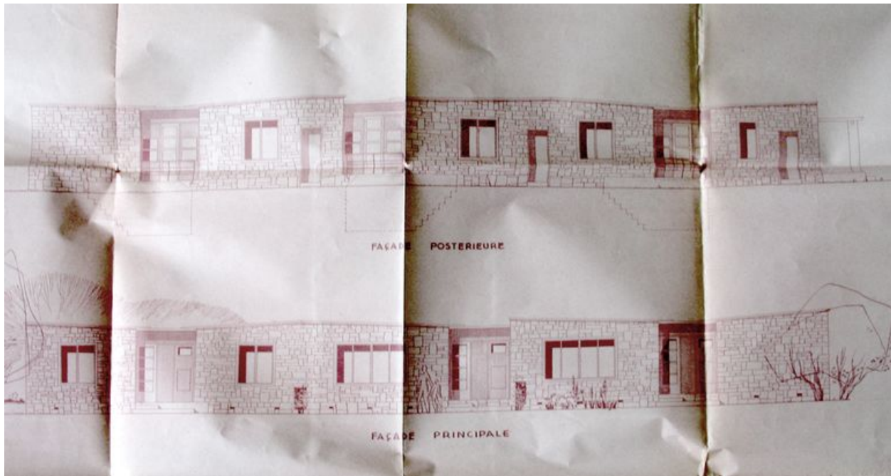
Élévation du bloc de trois maisons en rez-de-chaussée construites pour la cité du Vignolle, par Demaret et Moncet, 1953 (AC Montataire ; 102W4).
