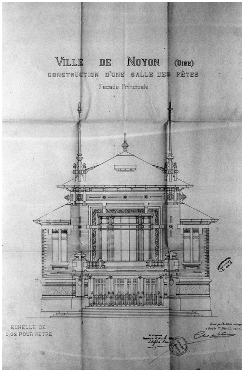
Élévation antérieure, projet par C. Letrosne, 1903 (AD Oise ; série O).
