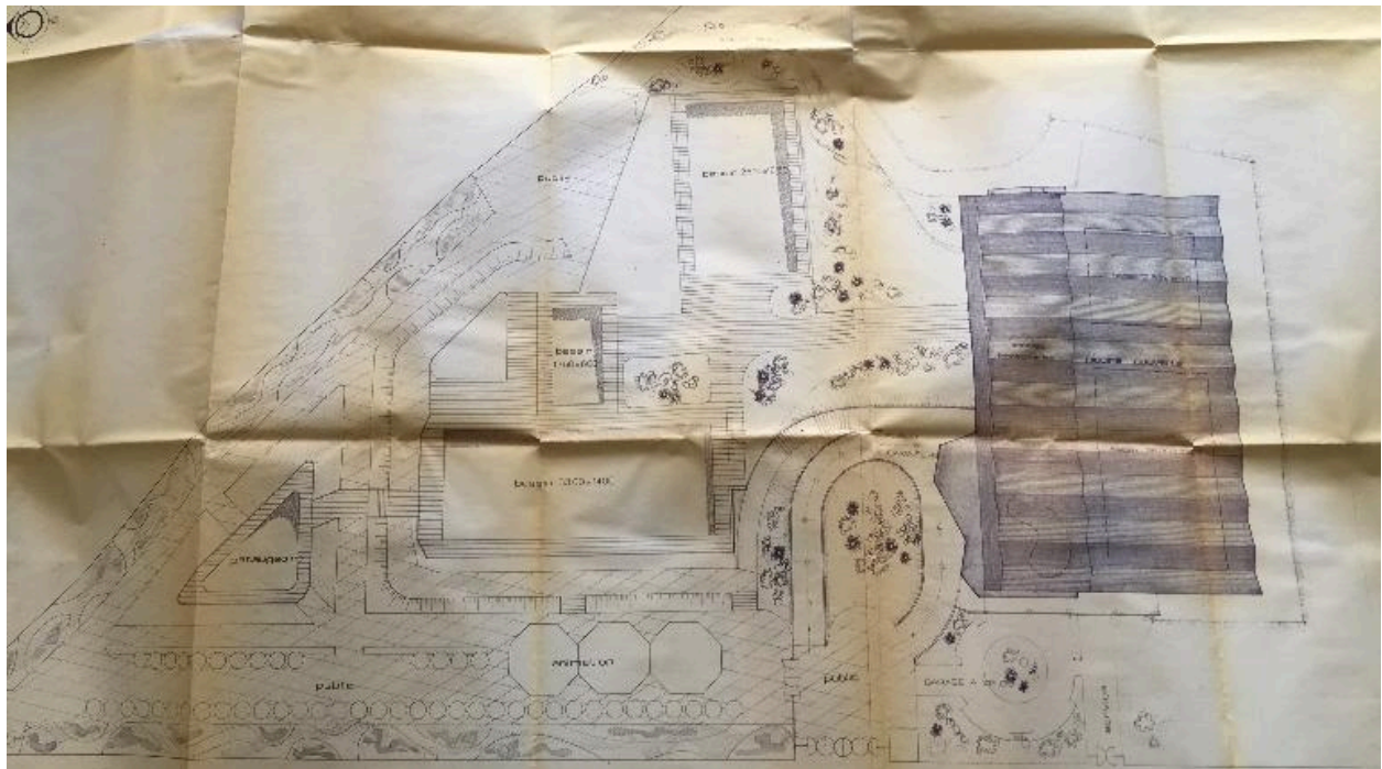
Plan masse de la piscine (ensemble des bassins extérieur et piscine couverte), projet de construction d'une piscine couverte, J. Doldourian architecte, 1973 (AC Soissons : 200 W 20).
