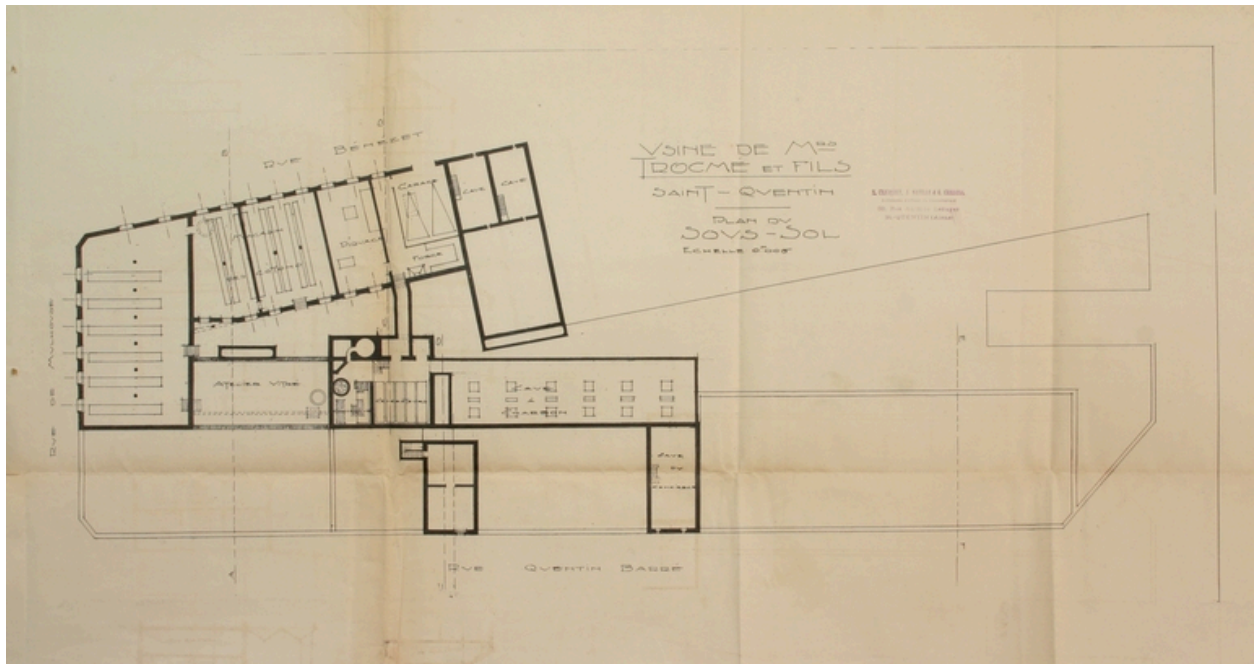
Plan des sous-sols de l'usine Trocmé à la veille de la Première Guerre mondiale dressé après 1919 par Chauquet, Navile et Christol (AD Aisne).
