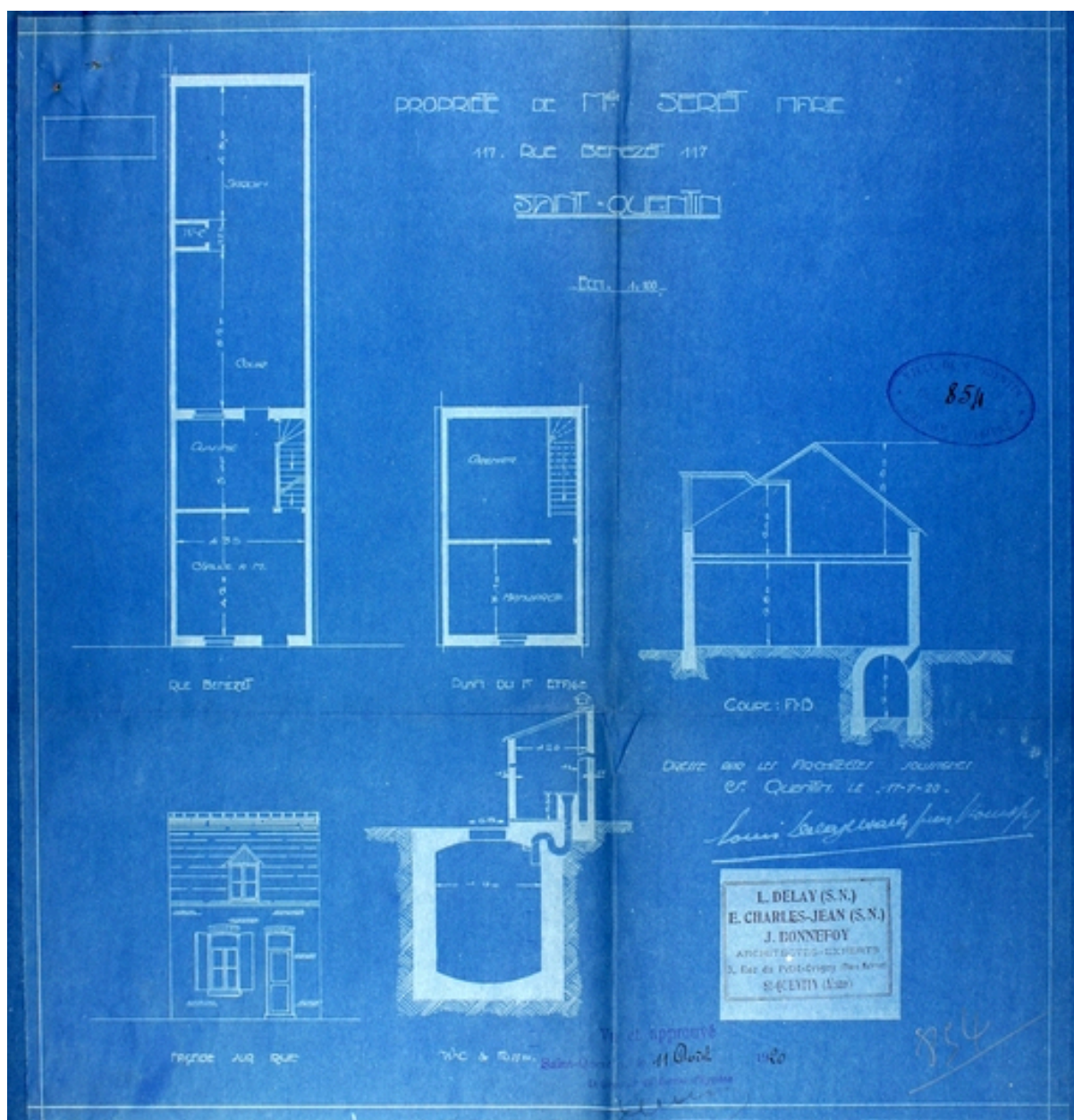
Plans d'une maison ouvrière, 1920 (AC Saint-Quentin).
