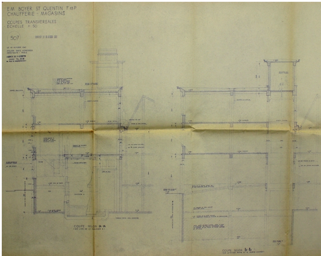
Coupes transversales de la chaufferie, par Honneger, 1947 (AC Saint-Quentin)..
