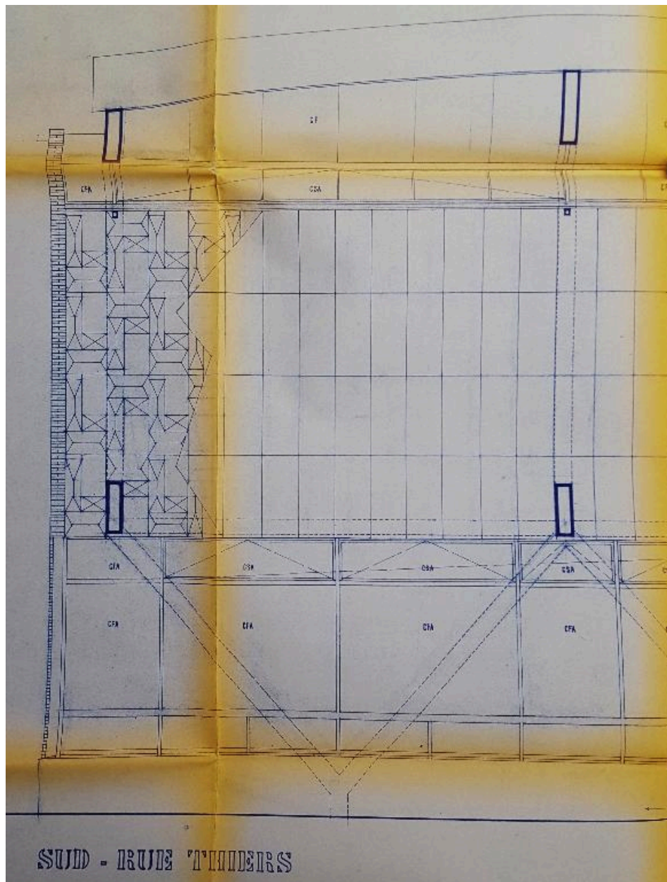
Détail du décor géométrique en fibrociment sur la façade sud, plan par Maurice Ego architecte, 1968 (AC Saint-Omer ; 3W40).
