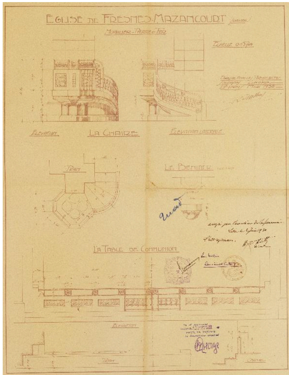
Mobilier pierre et fer (chaire, bénédicteur, table de communion), par R. Duthoit, mai 1930 (AD Somme ; 99 O 1846).
