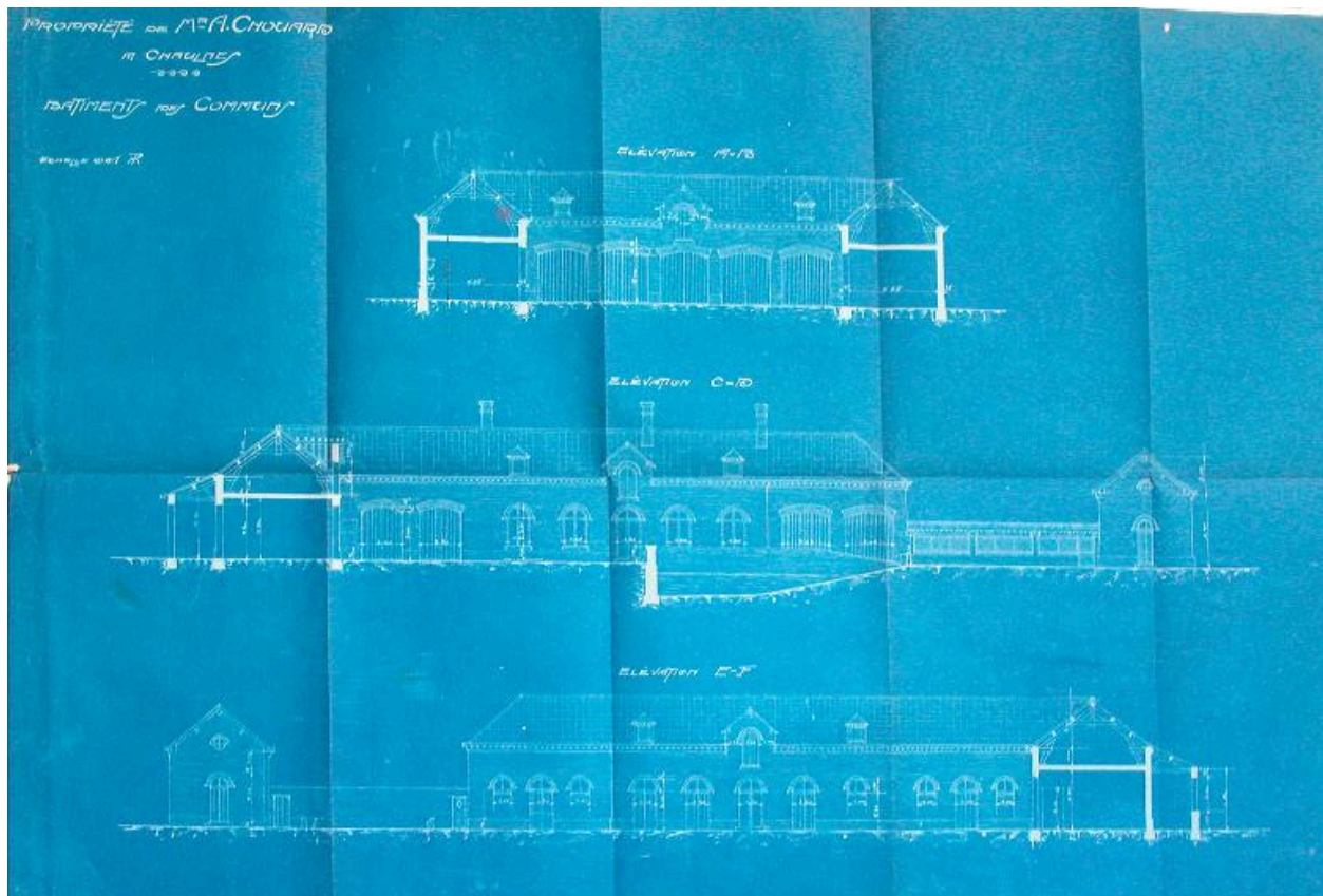
Propriété de Mr. A. Chouard. Chaulnes. Bâtiments des communes, élévations [Octave Lavoine architecte], [s.d.] (AD Somme ; 10 R 307.
