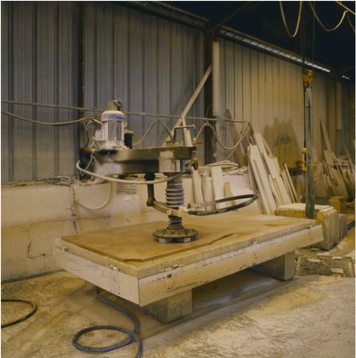
Machine à poncer la pierre (carrière Ouachée-Corpechot, Saint-Maximin).
