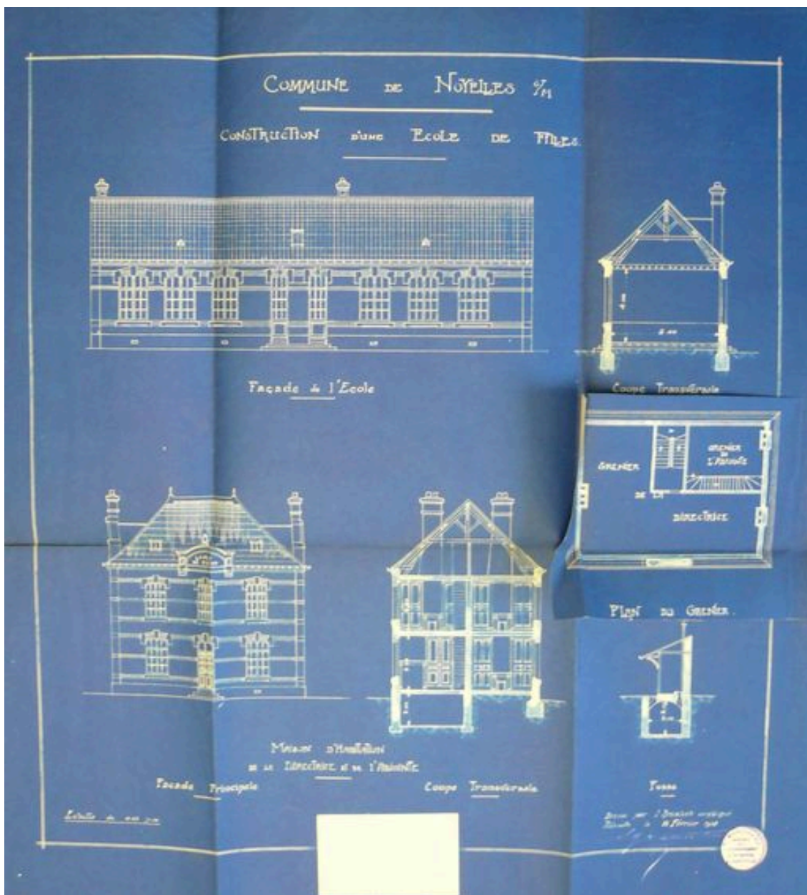
Projet de construction de la nouvelle école et de l'habitation de l'institutrice par Alfred Marchand, en 1913, plan, coupe et élévation.
