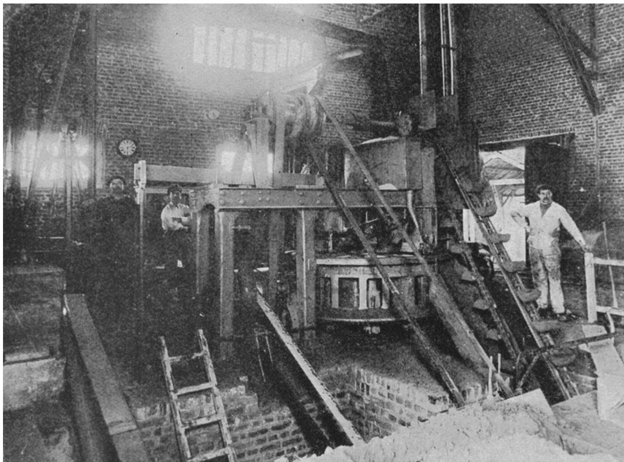
Presse rotative à briques, 1921 (Le Monde Illustré).
