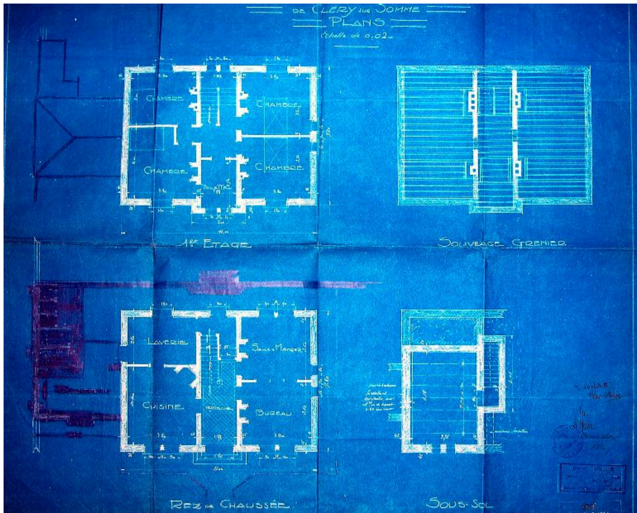
Plan du presbytère, 3e projet de reconstruction, Emmanuel Chainé (architecte), 1924 (AD Somme ; 99 O 1182).
