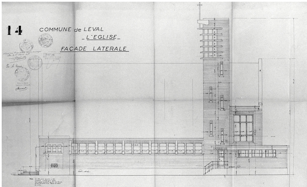
Elévation latérale de la nouvelle église ; plan 6 août 1958, Fernand Dumont (architecte communal). A.C. Leval : dossier église.
