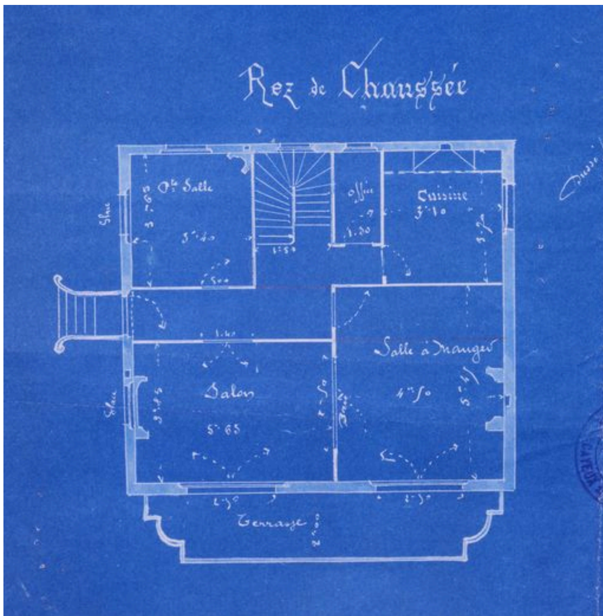
Plan du rez-de-chaussée, 1904 (AD Somme).
