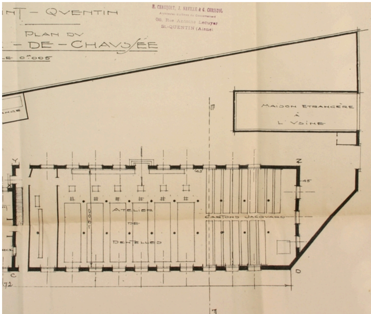
Plan du rez-de-chaussée de l'usine Trocmé à la veille de la Première Guerre mondiale, dressé après 1919 par Chauquet, Navile et Christol. Détail de l'atelier de dentelle (AD Aisne).
