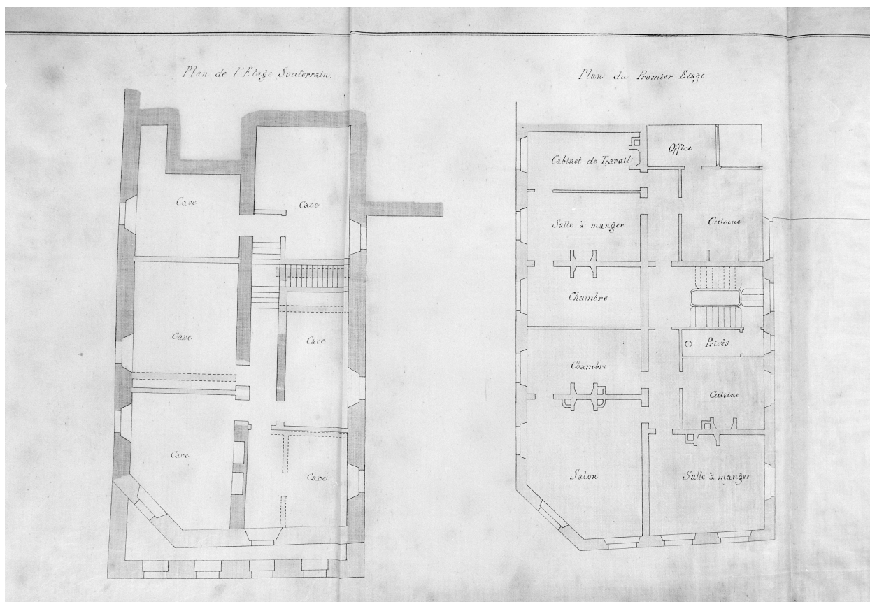
Presbytère, plan du 1er étage, du sous-sol (1881). A.D. Pas-de-Calais (2 0 - 1120).
