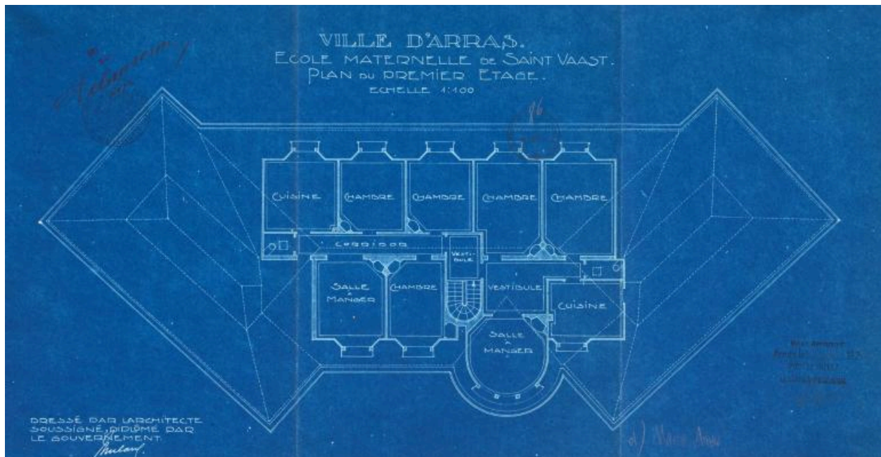
Ville d'Arras. École maternelle Saint-Vaast. Projet de reconstruction. Plan du premier étage, par Maurice Mulard architecte, vers 1922 (AD Pas-de-Calais ; 10R 4).
