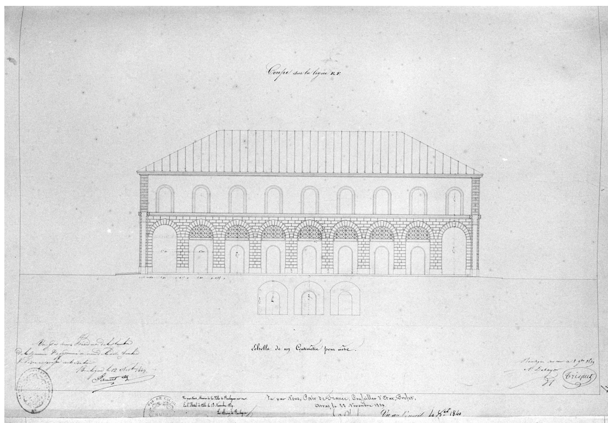
Douane, entrepôt public, coupe E-F, éch. 0,01 p.m. B.M. Boulogne-sur-Mer, ms 535 P. pl. 17.
